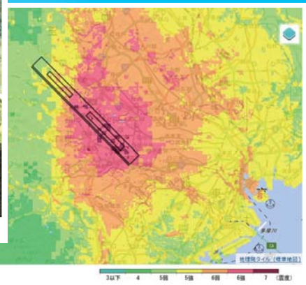
J-SHISの地震動予測地図(防災科研)
